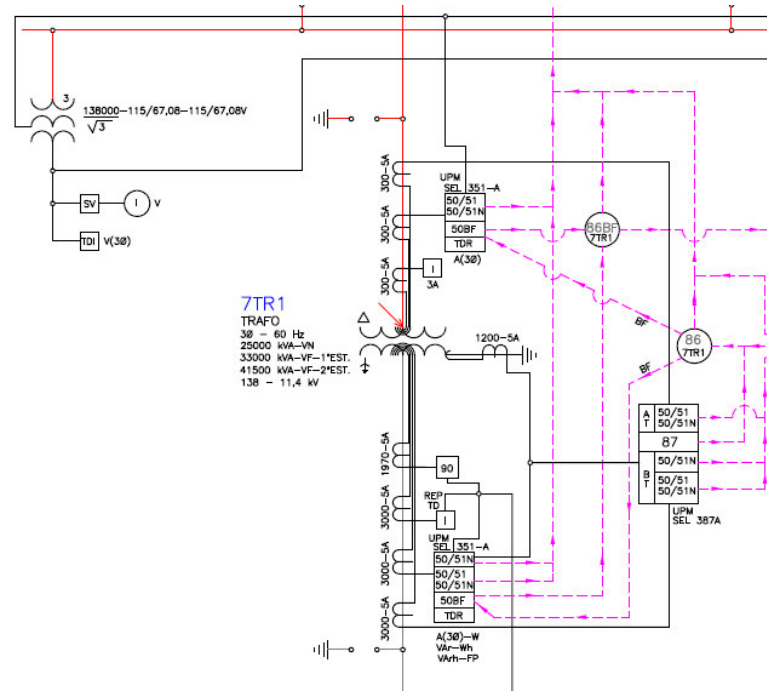
Figura 1 – Diagrama Unifilar do Transformador 7TR1
