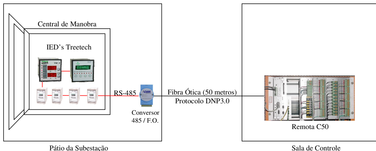
Figura 3 - Arquitetura do Sistema Descentralizado Adotado
